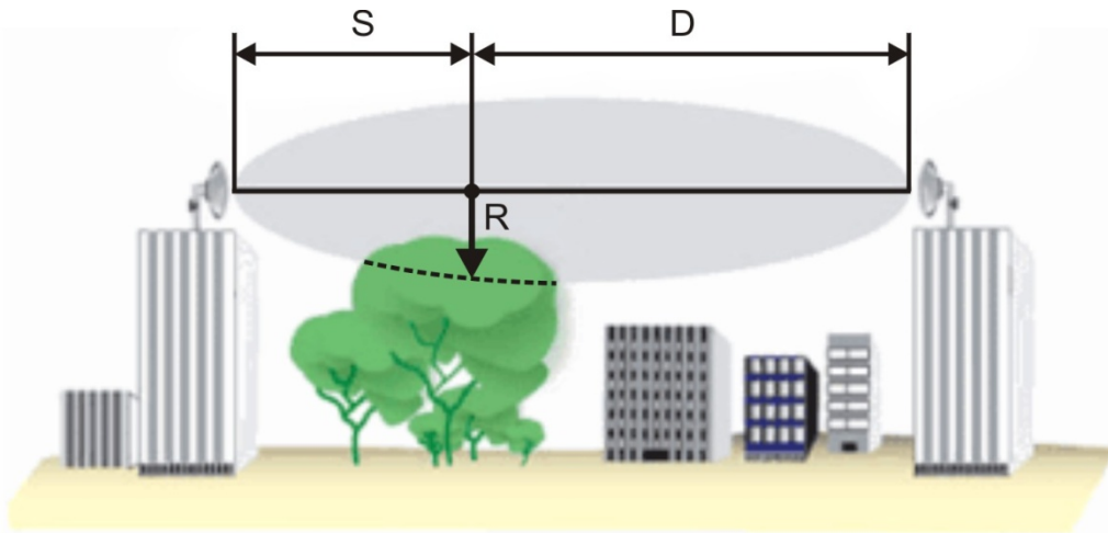
Рис. 3.5 Зона Френеля
