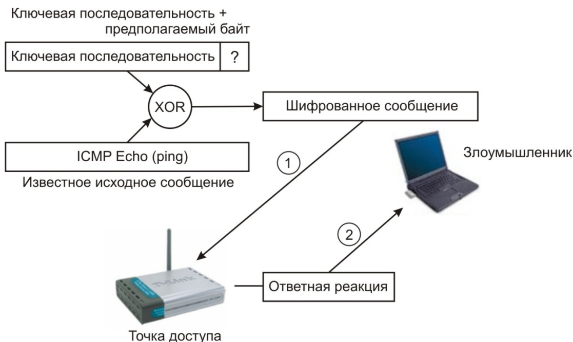
Рис. 2.15 «Выращивание» ключевой последовательности
